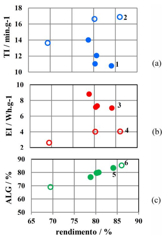
Figura 1 - Variaçã de (a) TI (b) EI e (c) ALG com o rendimento (círculos •/○, com/sem agitação)
